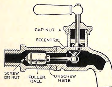
FIG. 2. FULLER-BALL FAUCET
